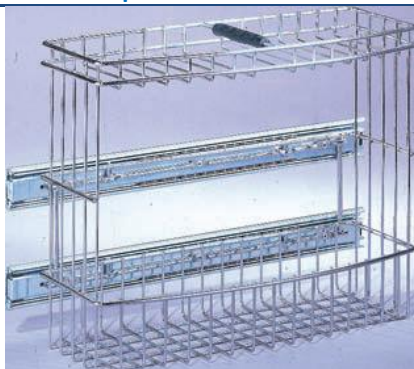
z.B. PROFILINE-DOUBLE-MASTER 40 DT und PROFILINE Drahtkorb passen in einen 60er Unterschrank
